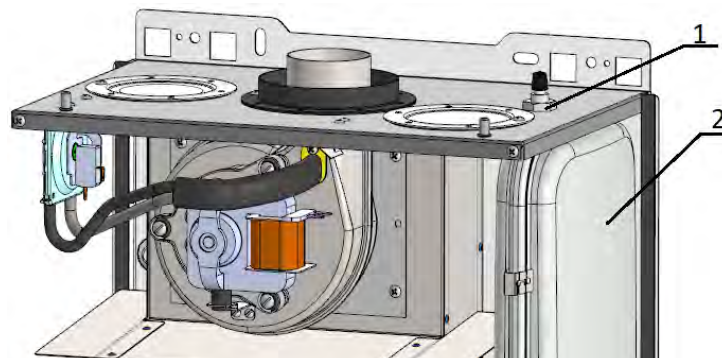
Рис. 17 Демонтаж расширительного бака
