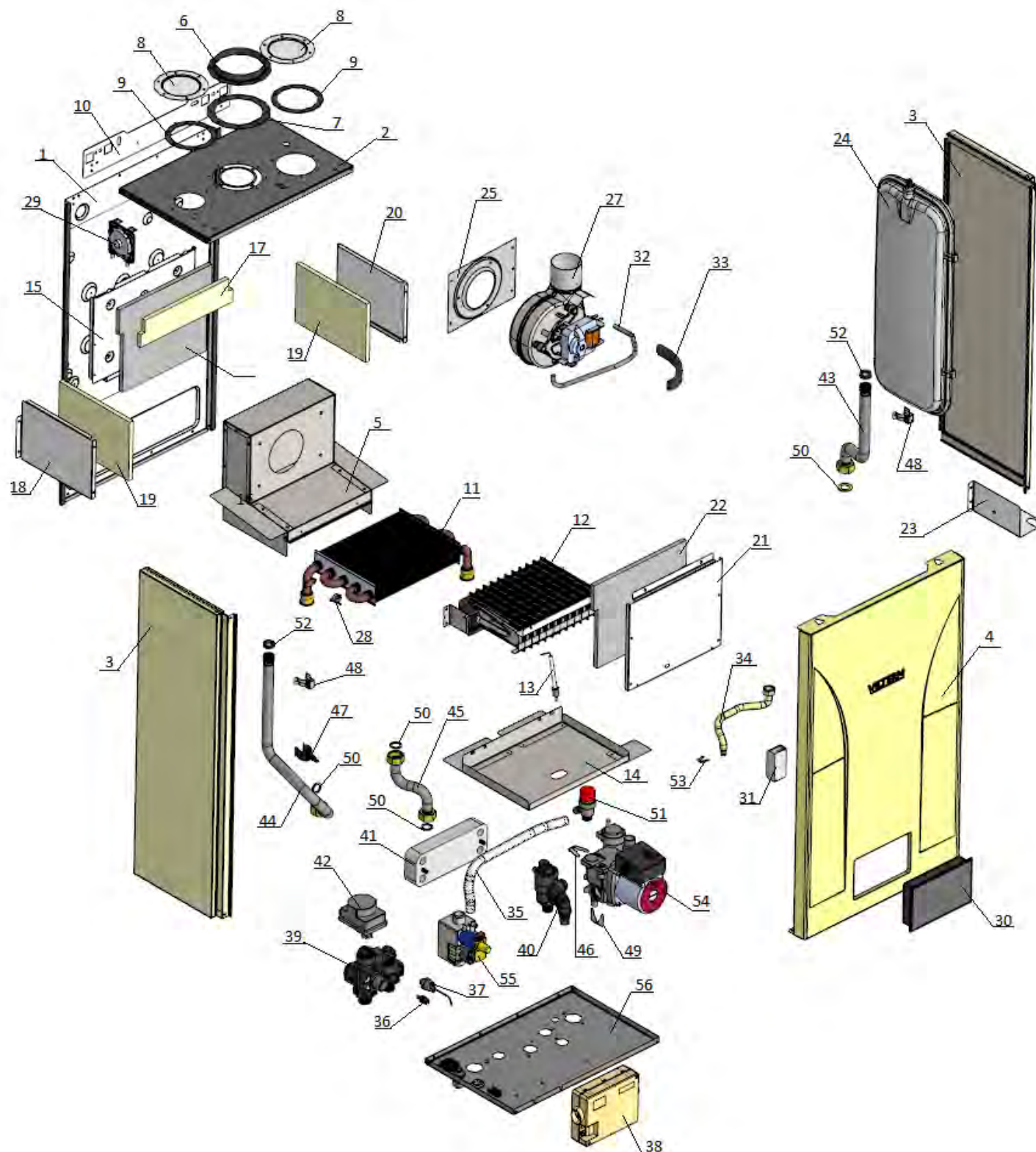
Рис. 19 Составные части котла
