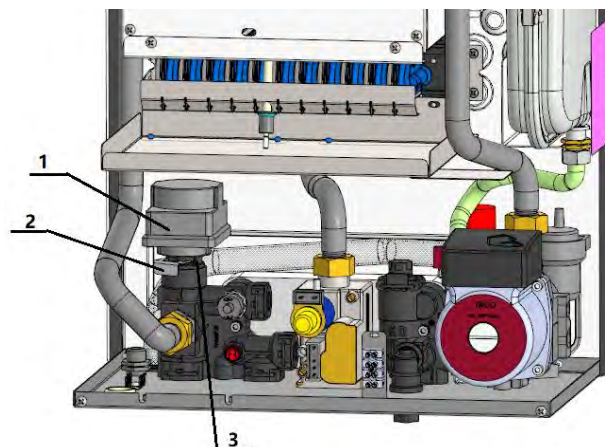
Рис. 14 Демонтаж трёхходового клапана
