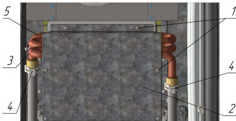
Рис. 10 Демонтаж теплообменника
