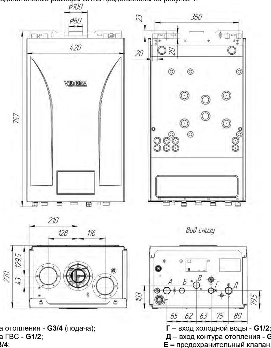
Рис. 1 Габаритные и присоединительные размеры котла
