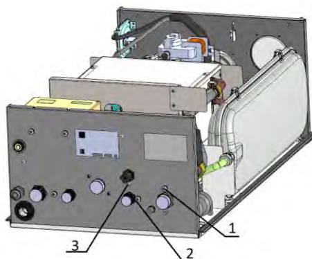
Рис. 12 Демонтаж гидроблока
